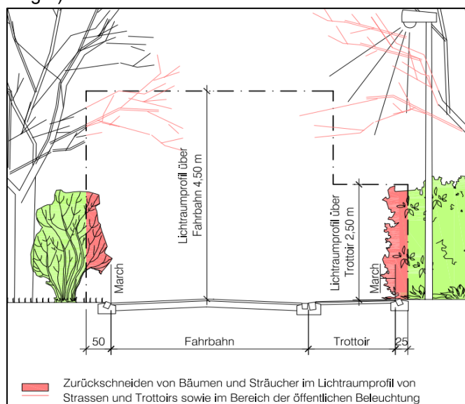
Abbildung 1, Lichtraumprofil Strasse
